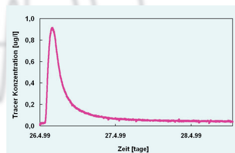
Eosindurchgang im Grundwasser
